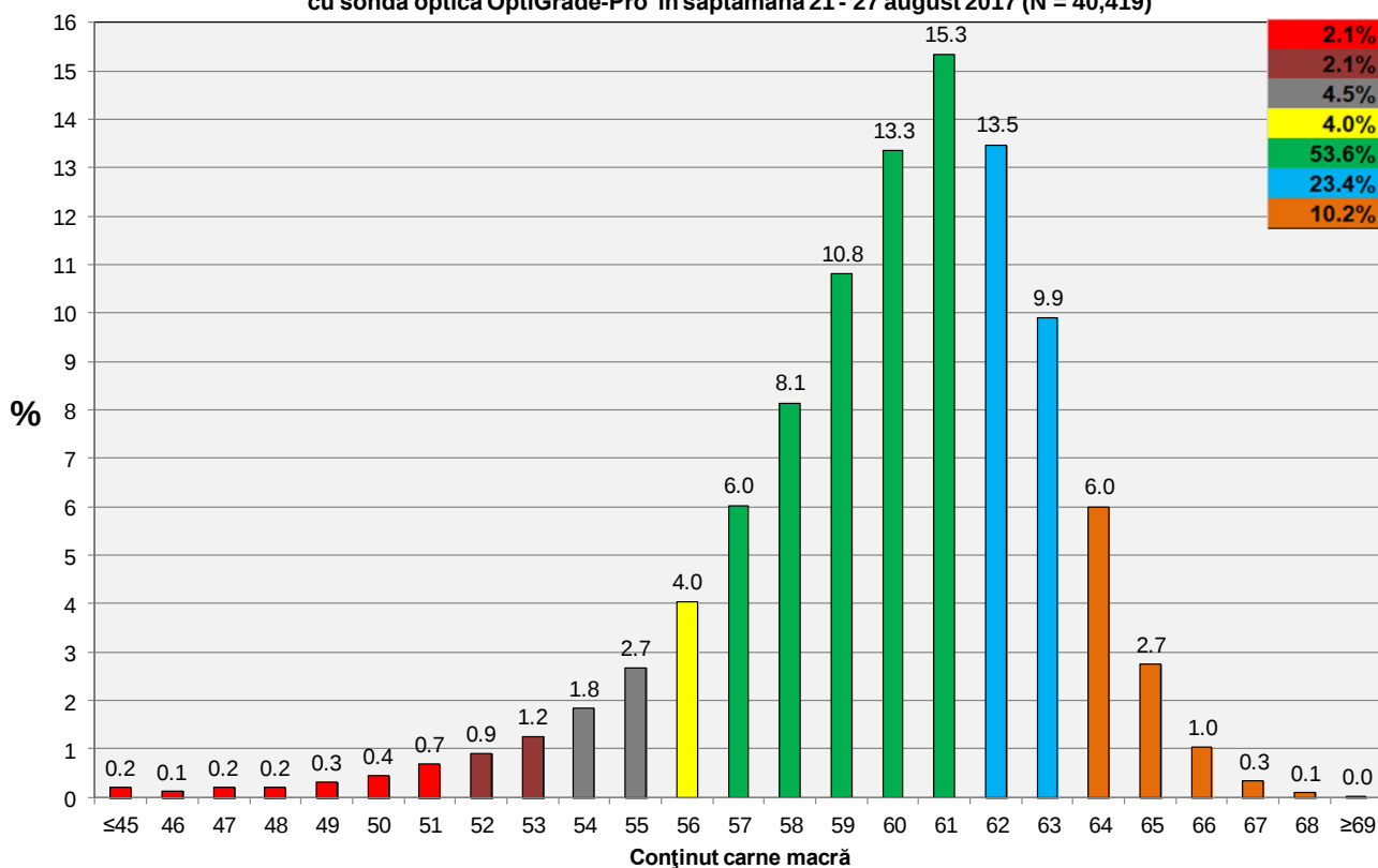
Distribuția conținutului de carne macră a carcaselor clasificate în România cu echipamentul cu sondă optică OptiGrade-Pro în săptămâna 21 - 27 august 2017 (N = 40,419)
