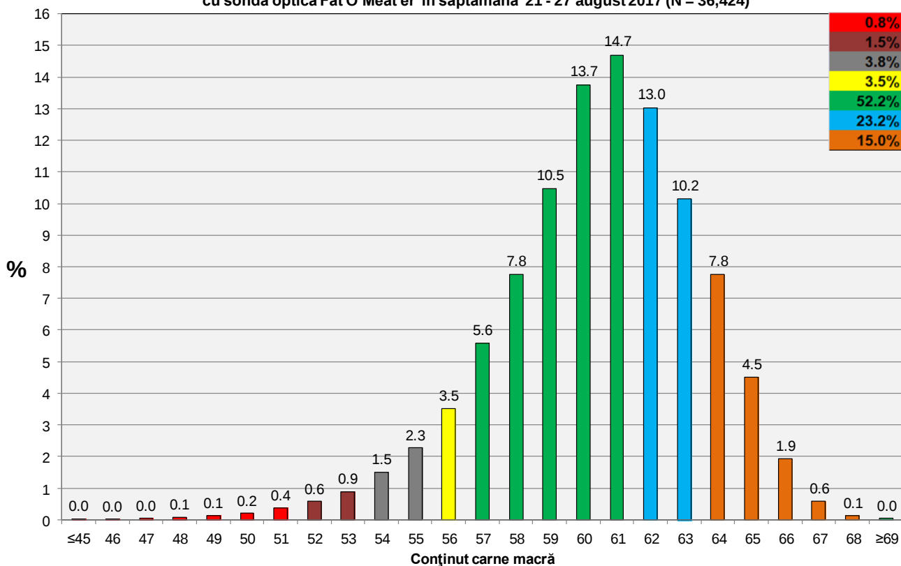
Distribuția conținutului de carne macră a carcaselor clasificate în România cu echipamentul cu sondă optică Fat O Meat'er în săptămâna 21 - 27 august 2017 (N = 36,424)
