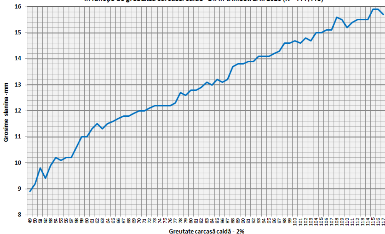
Grosimea slaninii cu echipamentul cu sondă optică OptiGrade-Pro în România în funcție de greutatea carcasei calde - 2% în trimestrul III 2025 (N = 777,118)
