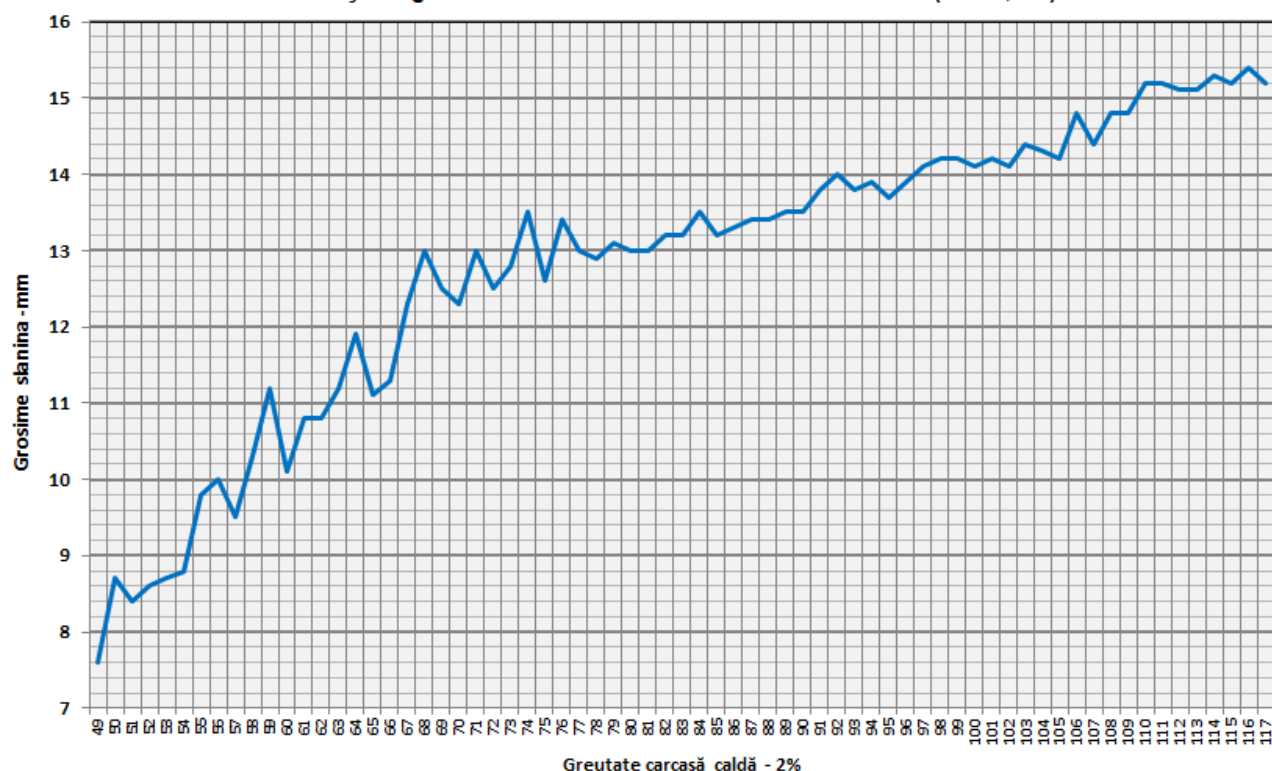
Grosimea slaninii cu echipamentul cu sondă optică Fat-O-Meater în România în funcție de greutatea carcasei calde - 2% în trimestrul III 2025 (N = 45,121)
