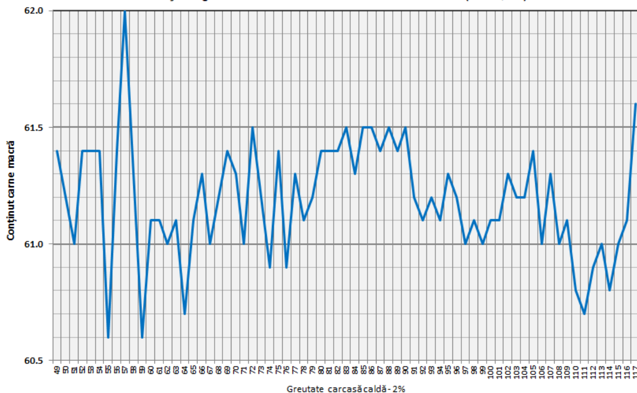
Conținutul de carne macră cu echipamentul cu sondă optică Fat-O-Meater în România în funcție de greutatea carcasei calde - 2% în trimestrul III 2025 (N = 45,121)
